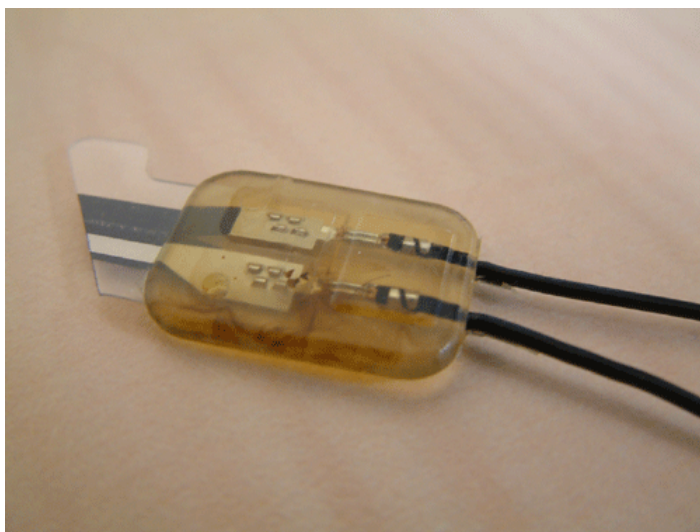
Connexion flex-fil renforcée par surmoulage
